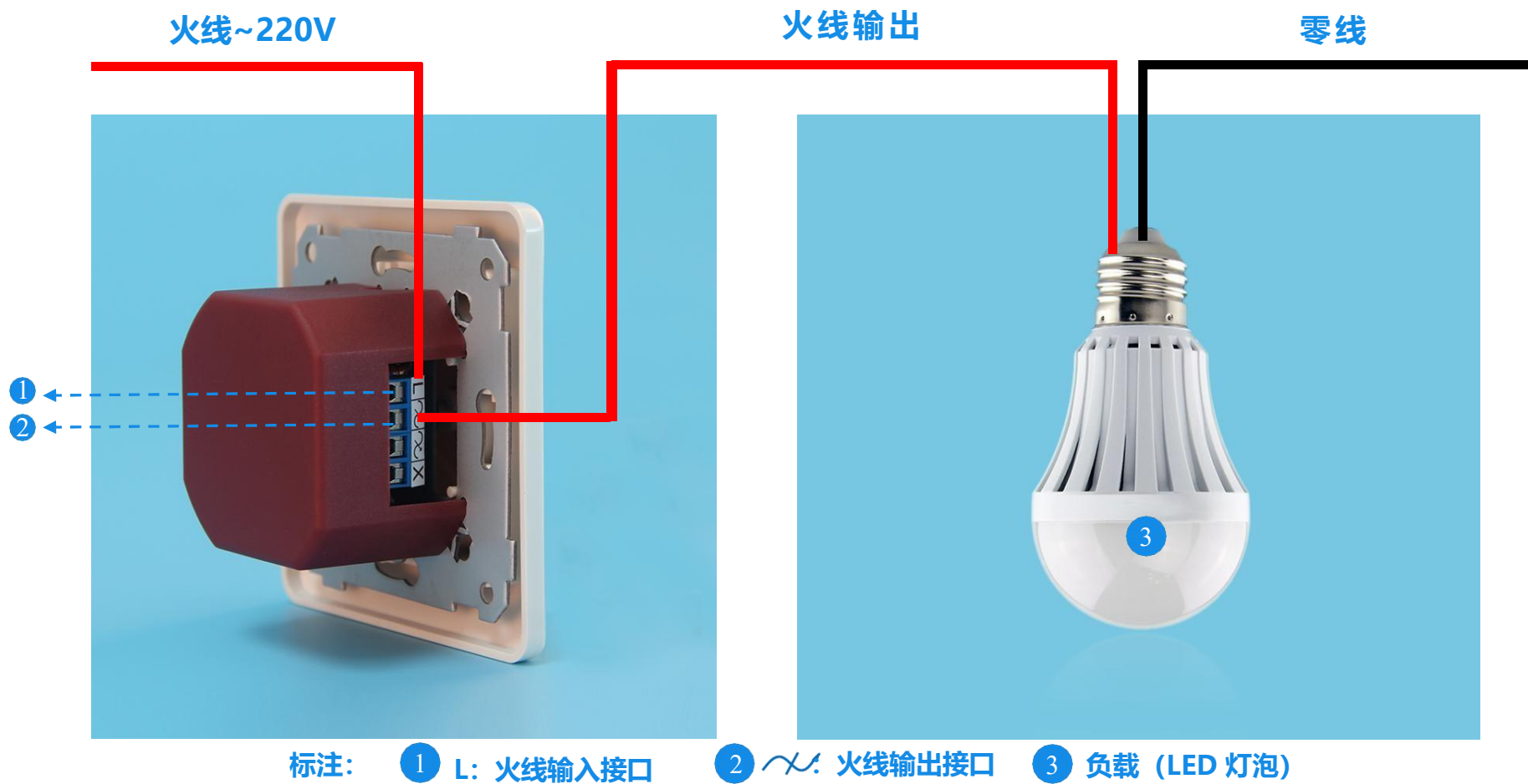
单控接线示意图
