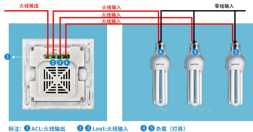
BRT-110/114 接线示意图
