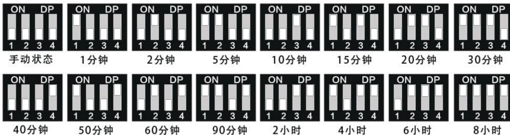
BRT-111A/115A 拨码调节示意图
