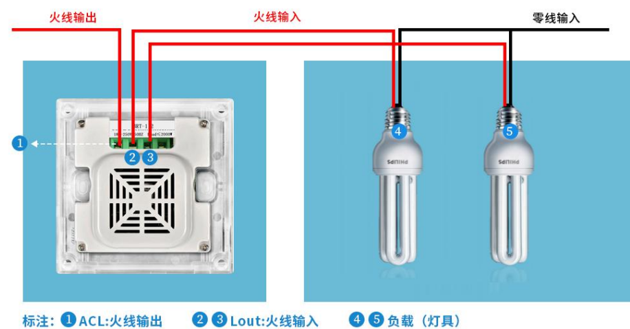
BRT-109/113 接线示意图
